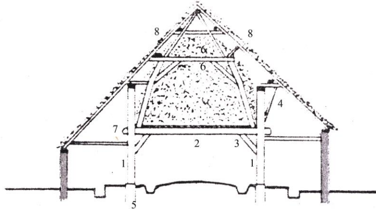
Driebeukig hallehuis. 1 stijl, 2 ankerbalk, 3 korbeel, 4 schoor, 5 poer, 6 kaspant, 7 oor en 8 gording (Huijts, 1995)
