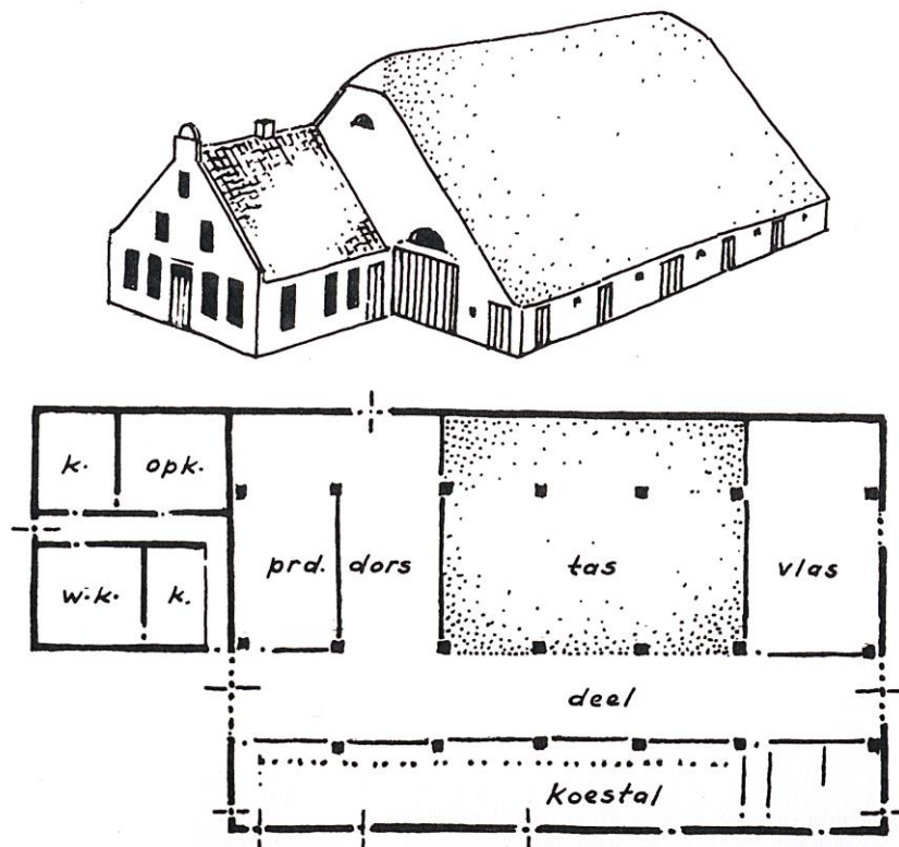
Tekening van een boerderij van het Vlaamse schuurtype (afb. 18 Hekker, 1986)
