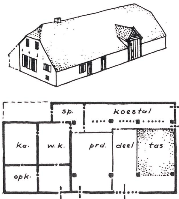
Tekening van de Overmase dwarsdeelboerderij Voordijk 406 (afb. 16 Hekker, 1986)
